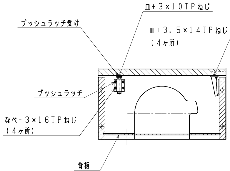
B-B断面
