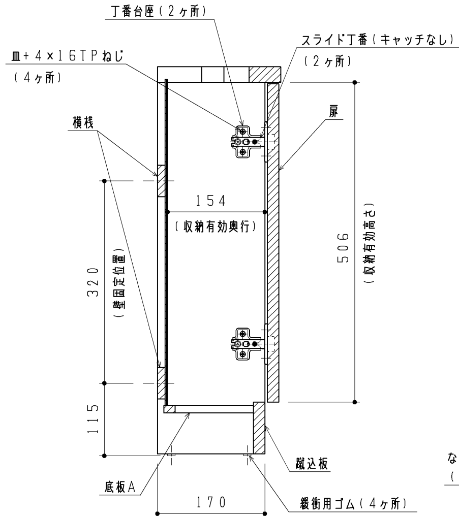
A-A断面
