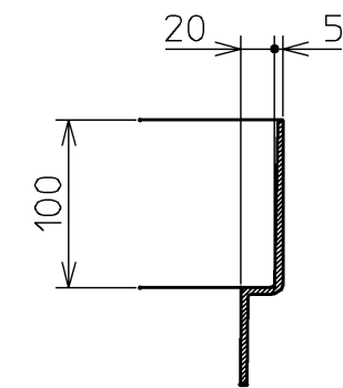
壁のせ部(防水リム部)詳細
