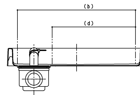
断面B-B
