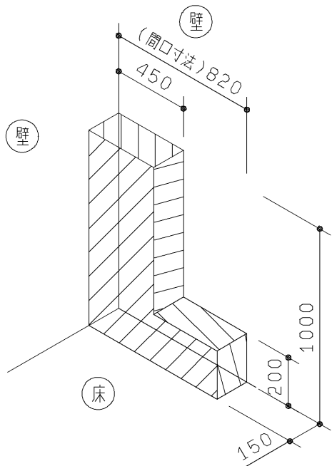
左図と異なる位置から配管を取り出す場合
