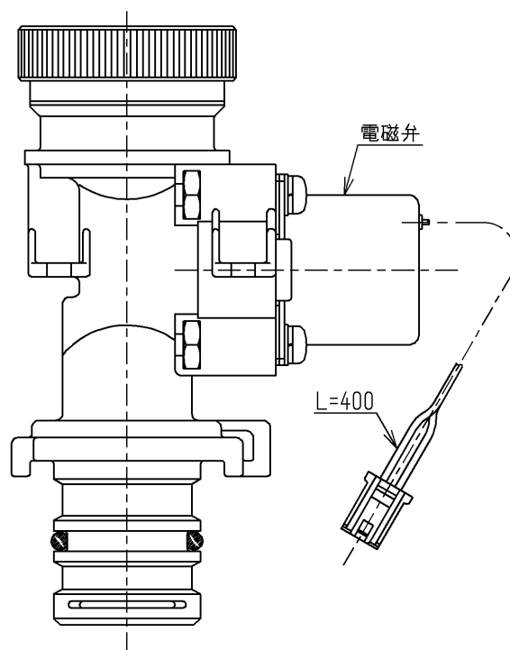
駆動部
