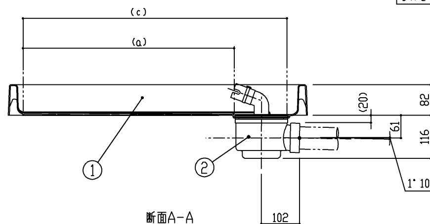
洗濯機設置有効寸法組合せ
