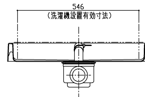
断面B-B
