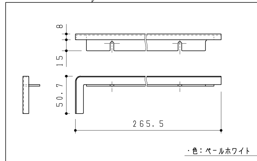
天板キャップL
