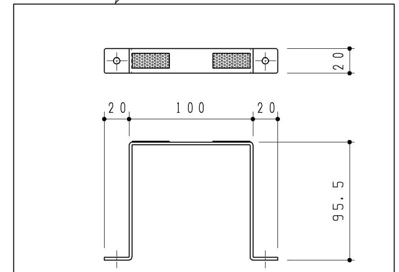
カウンター支持金具セット
