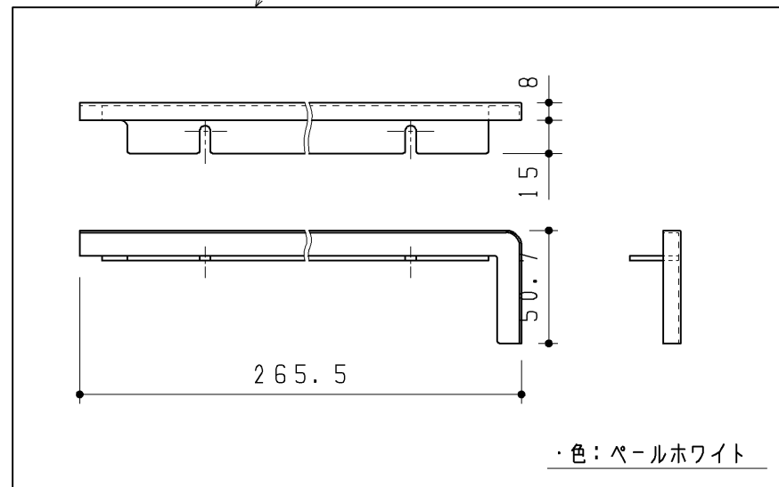
天板キャップR
