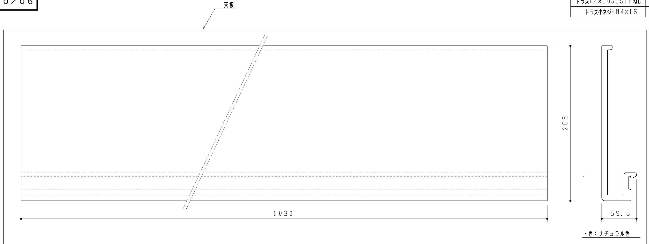
天板キャップR
