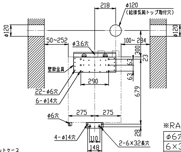
■壁取付位置（1:20）
