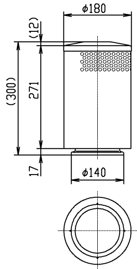
■ 排気トップ (別売品: RAE16P)
