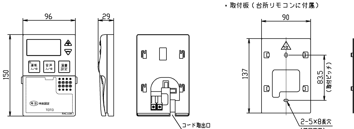
■ 台所リモコン (別売品: RAC110KT) (1:5)
