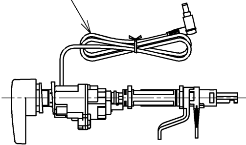
便器洗浄コード L=1500
