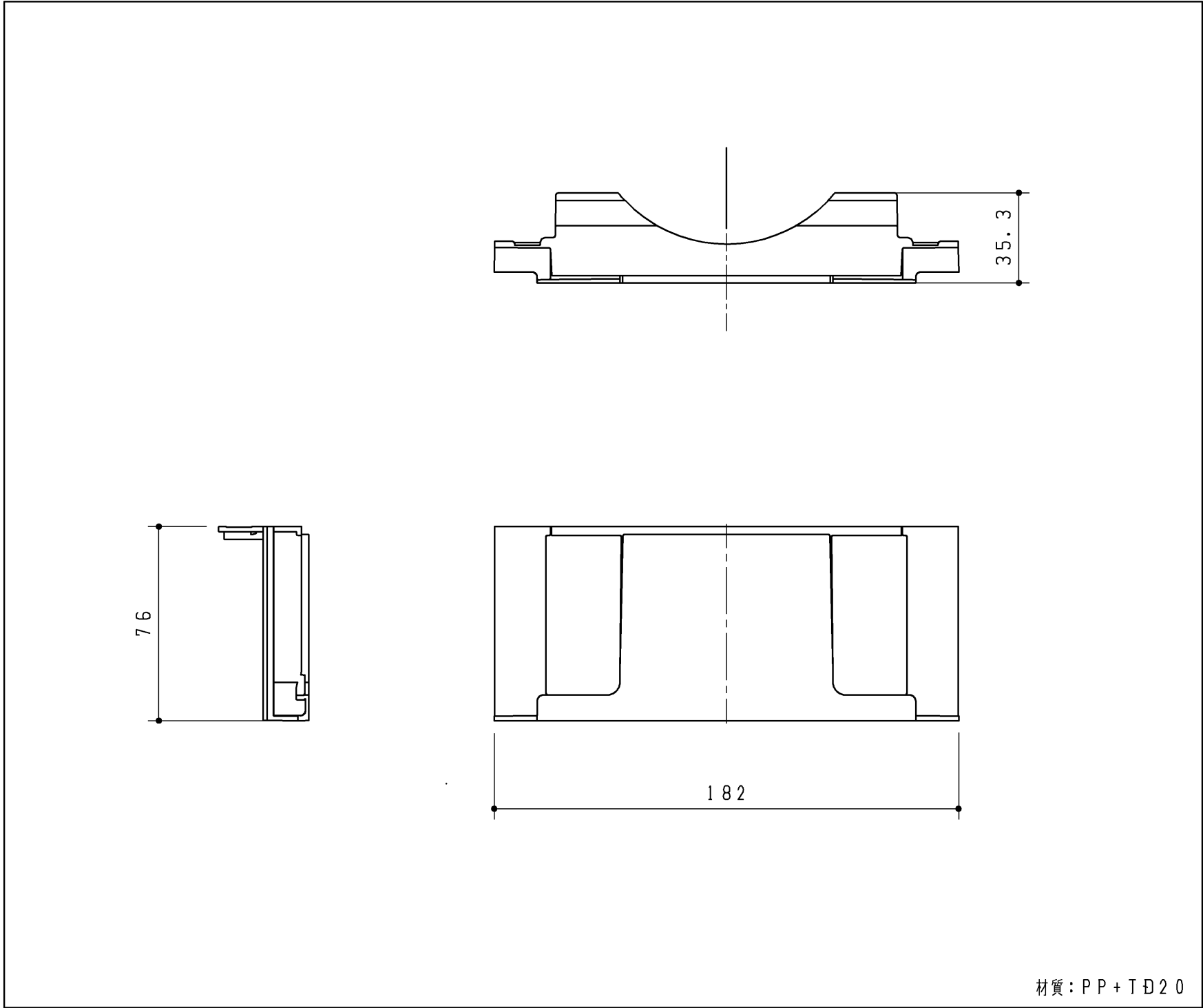
カバー（配管）
