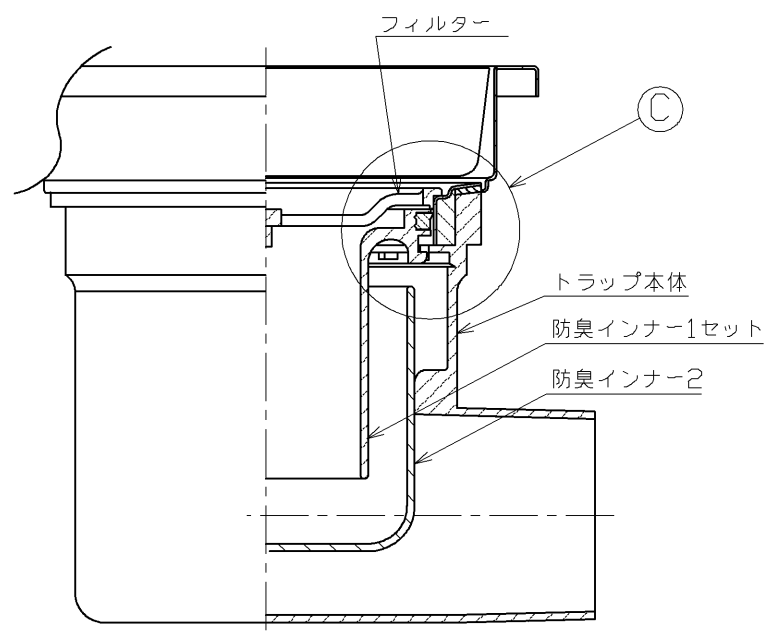
トラップ詳細図(1:2)
