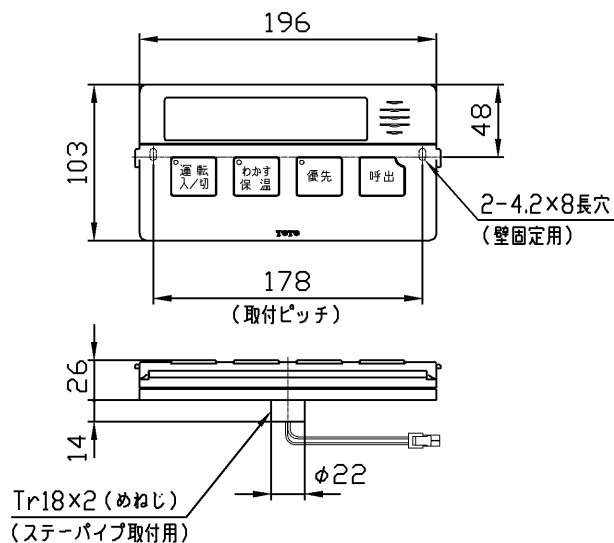
■浴室リモコン（別売品：RAC147F） ※ステーパイプ、カセットケースは浴室用屋外カバーセット（1：5）
