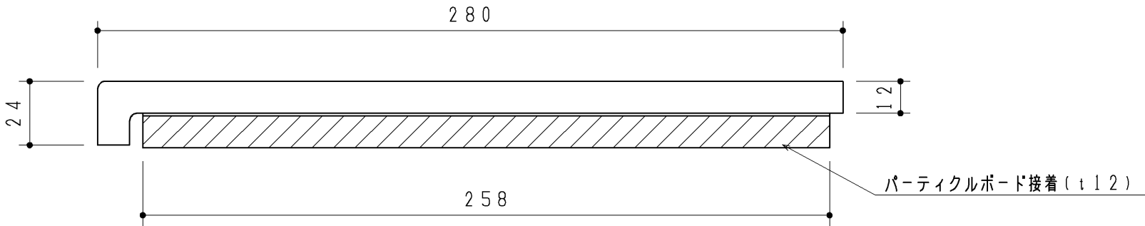
A-A断面図 (S=1:2)
