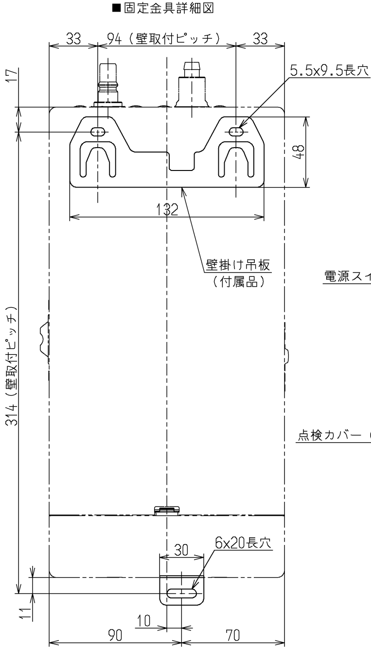
■固定金具詳細図
