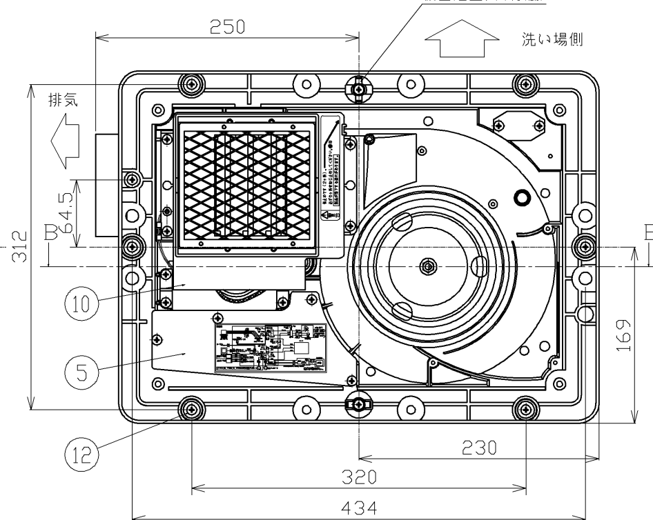
天井取付図 (1:5)
