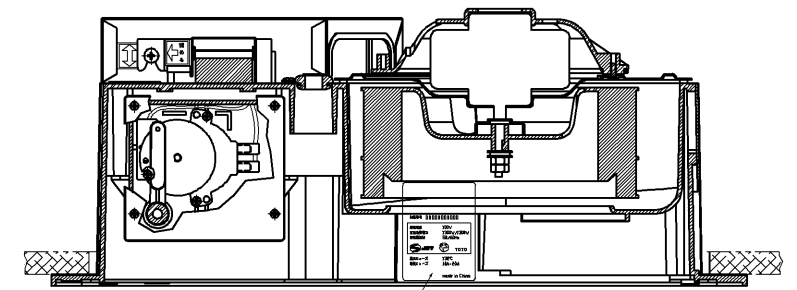
B-B断面
