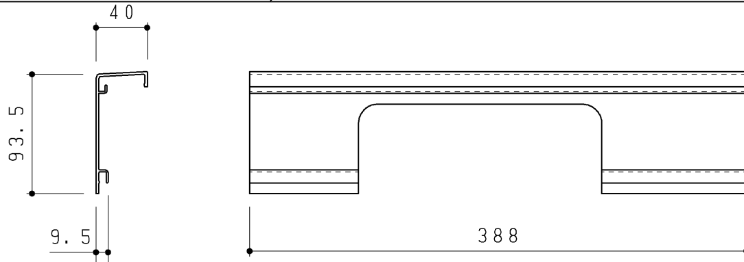
配管カバーL（間口小）（ホワイト）
