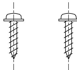
座金付なベタッピンねじφ4×18
