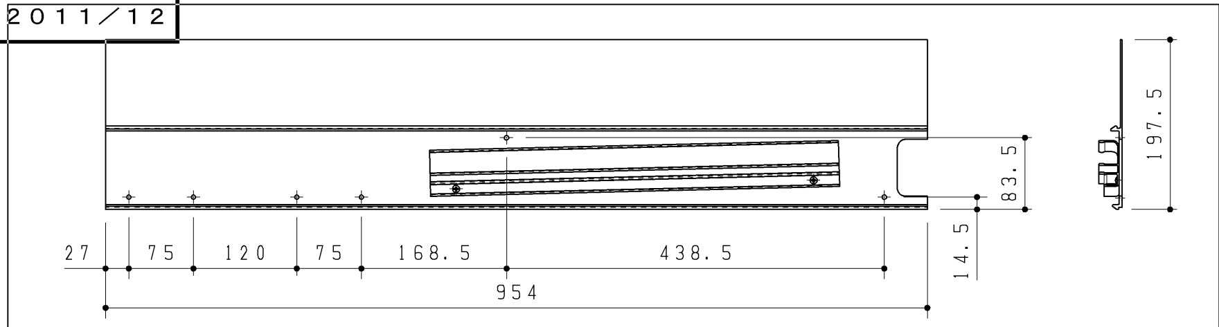
配管カバー
