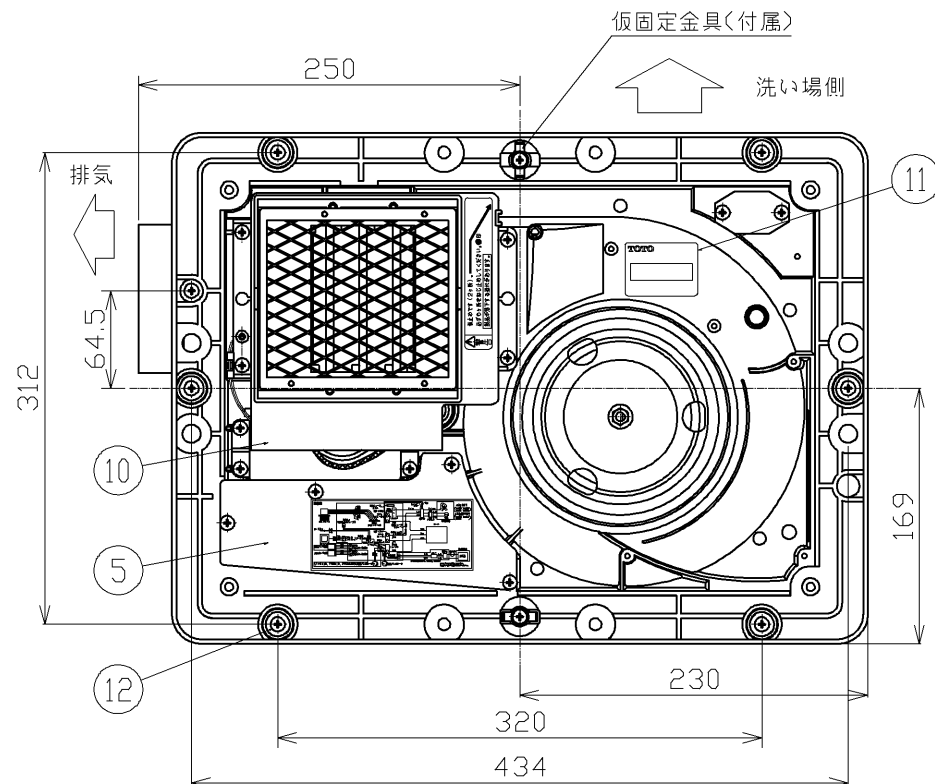
天井取付図 (1:5)
