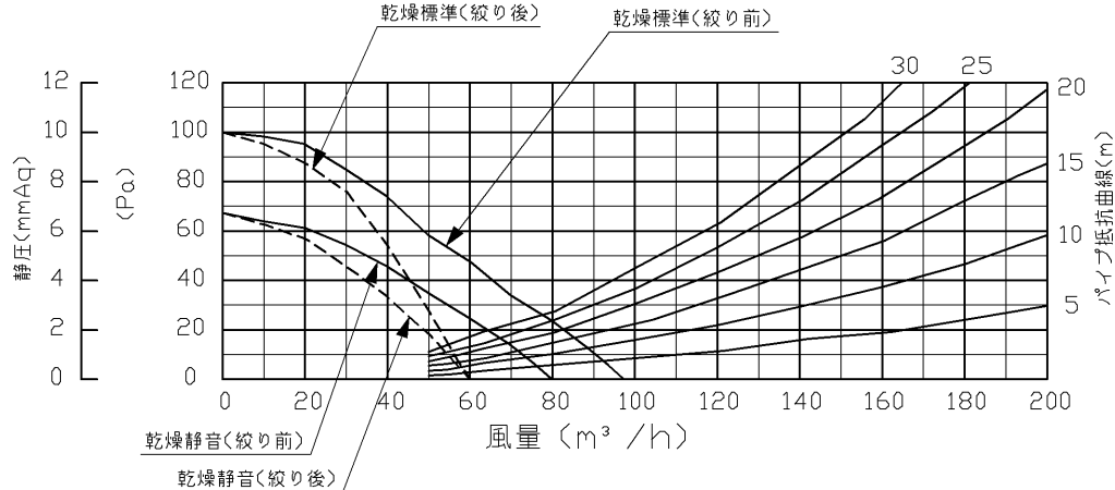
静圧風量特性曲線(乾燥運転時)
