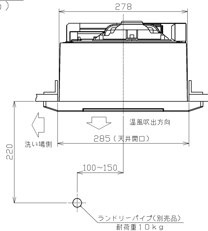
A-A断面
