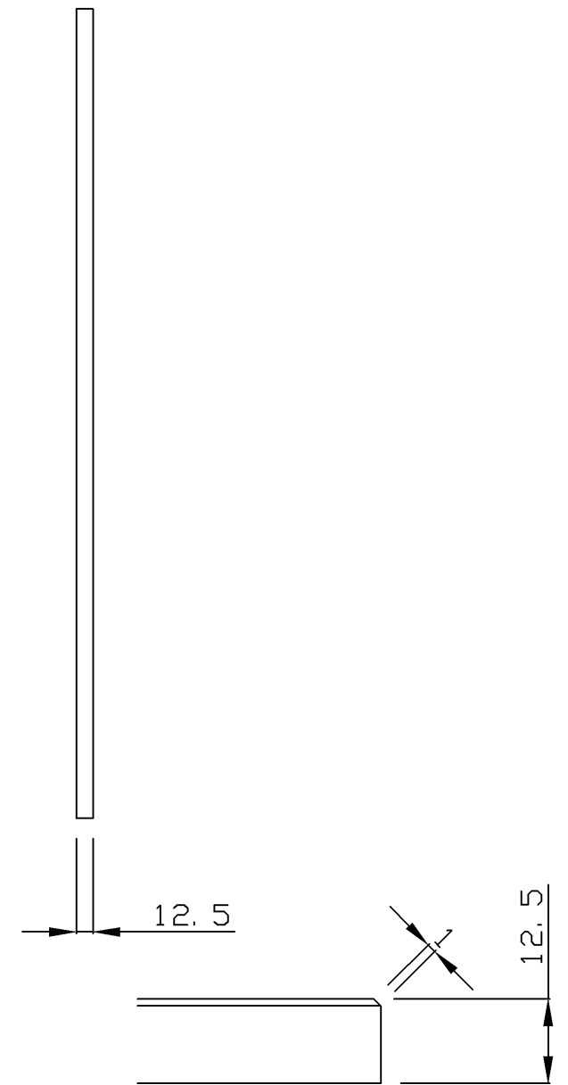
A部（面取り部）拡大図
