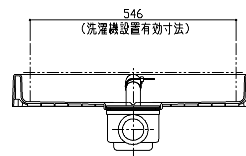
断面B-B
