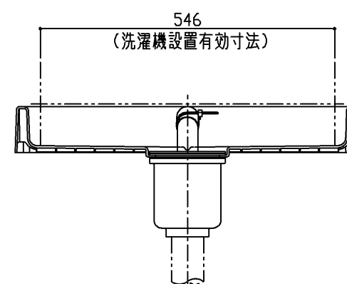
断面B-B
