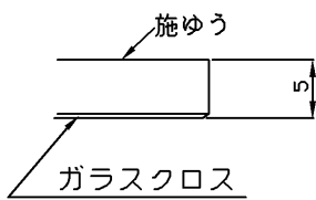
B部（断面部）拡大図 ※長辺1辺以外の3辺
