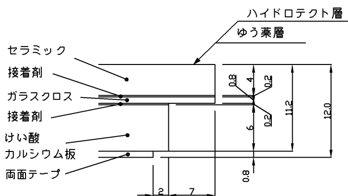
A部（断面図）拡大図2：1
