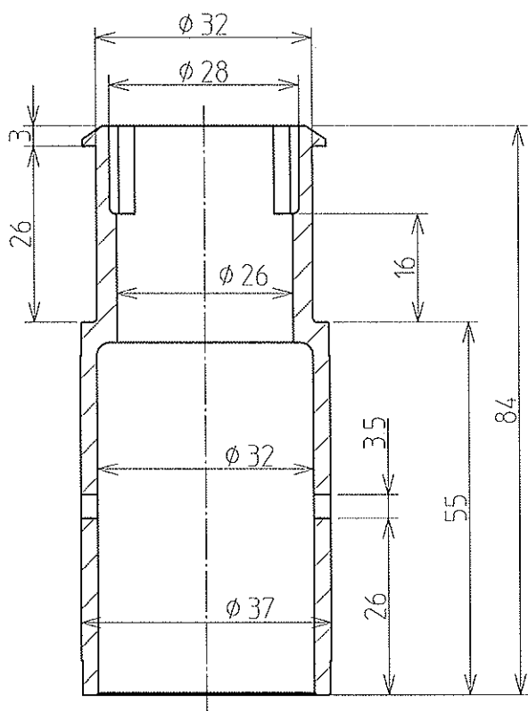
A-A断面
