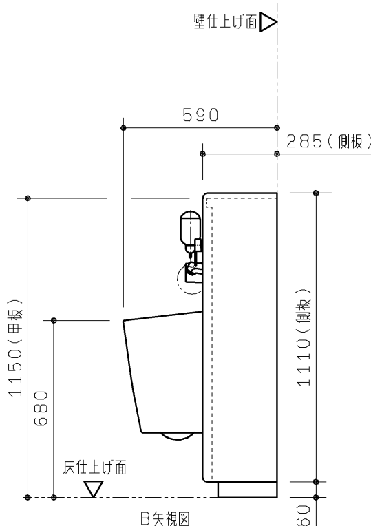
B矢視図
