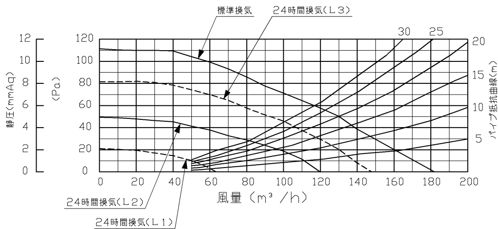
静圧風量特性曲線（換気運転時）
