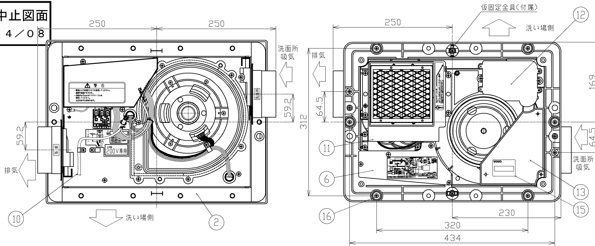
天井取付図 (1:5)
