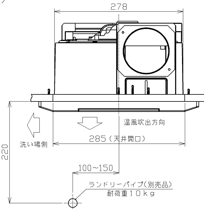
A-A断面
