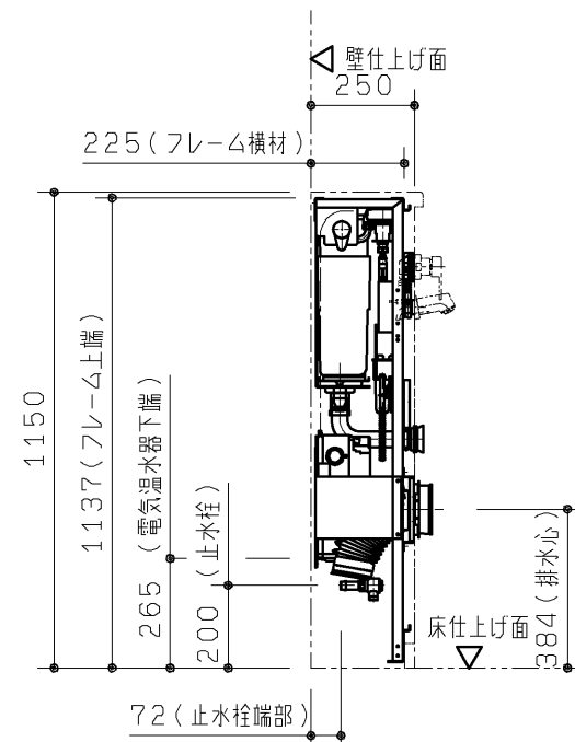
尺視圖
