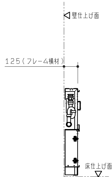
戸视图
