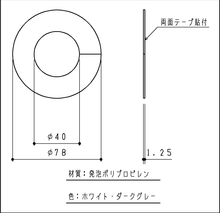
カバー（1ヶ）
