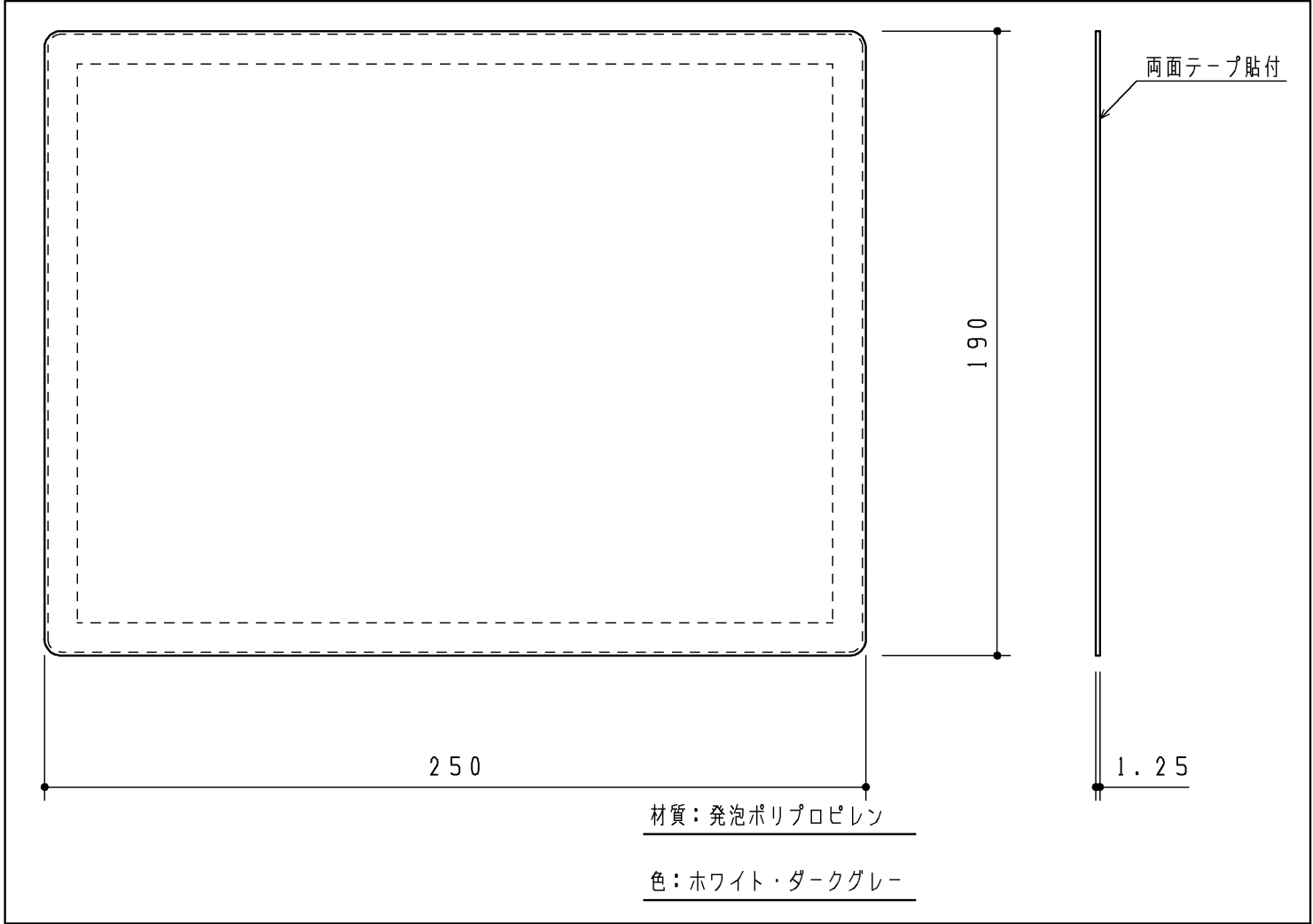
カバー組品（1ヶ）
