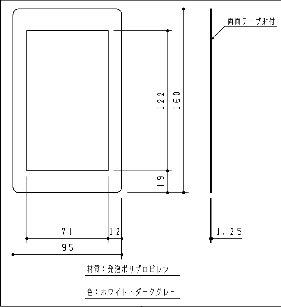
カバー（コンセント）（1ヶ）
