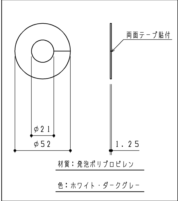
カバー（1ヶ）
