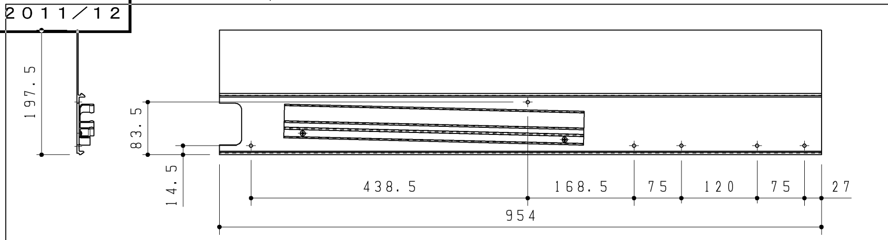
配管カバー
