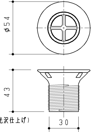
排水金具
