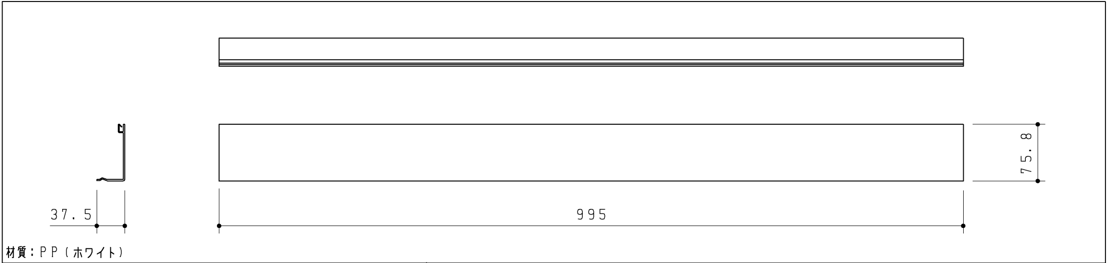
配管カバー
