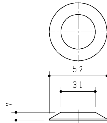
材質：EPDM (黒) 尺度： 1 : 2
