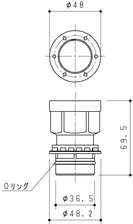
材質：PP (ホワイト) + EPDM (黒) 尺度： 1 : 2
