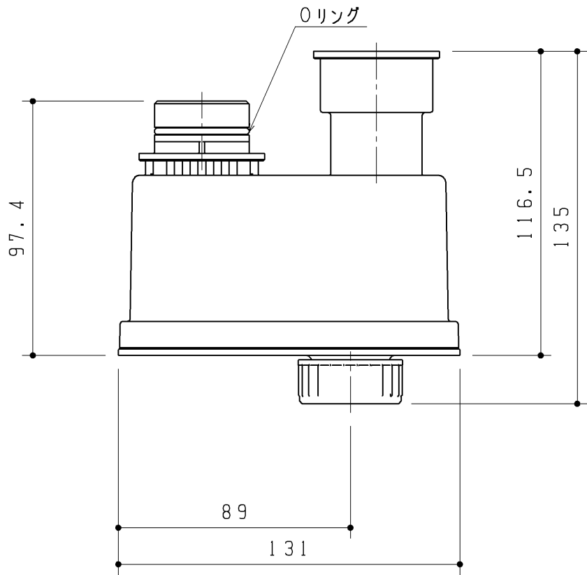
材質：PVC (アイボリー) + EPDM (黒) 尺度： 1 : 2
