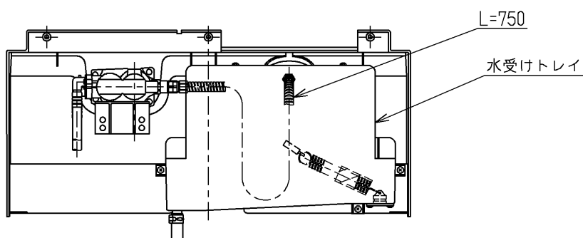
裏面図
