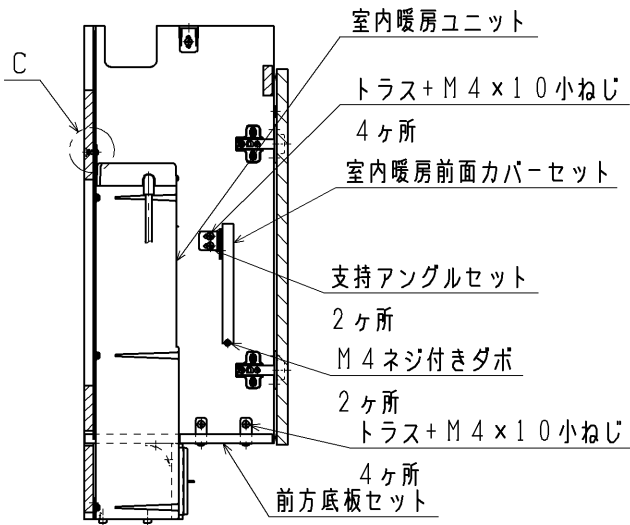
室内暖房ユニット固定詳細
