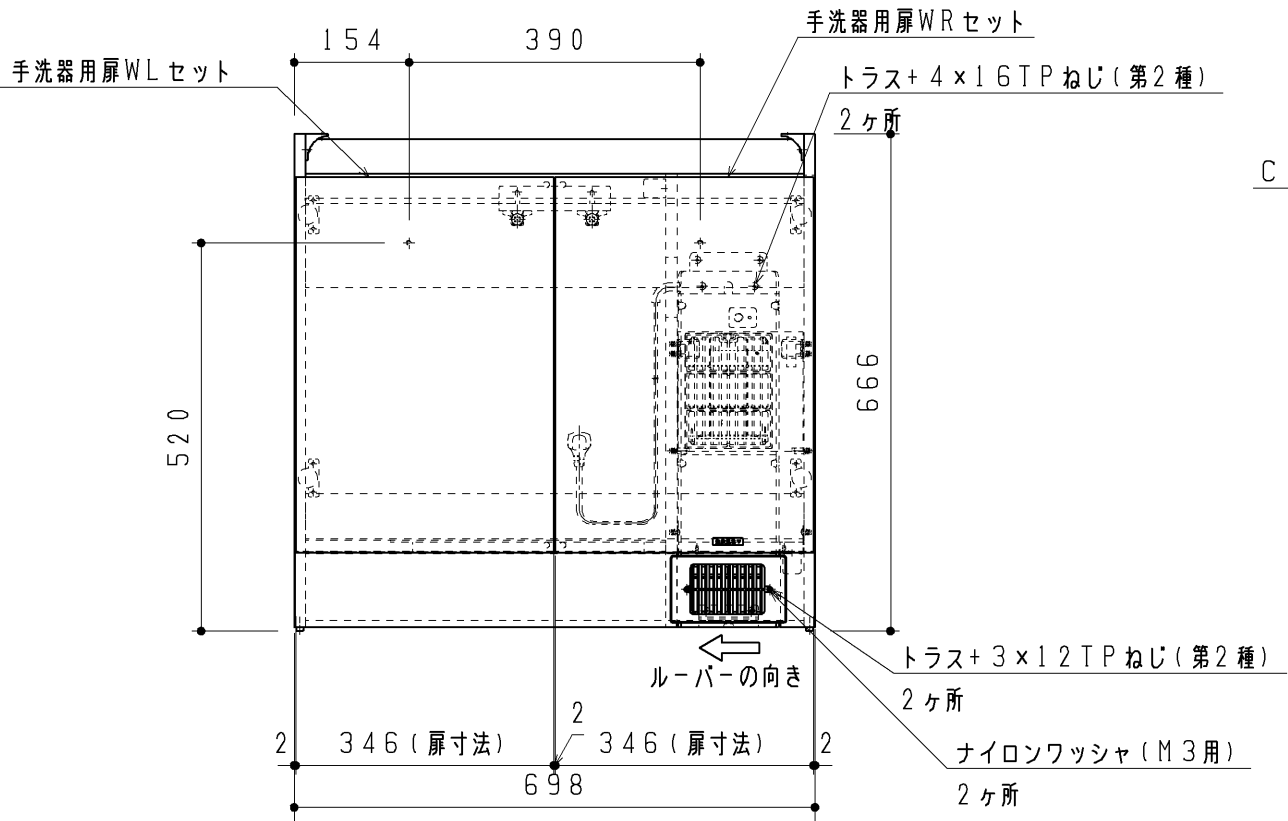
室内暖房ユニット固定詳細
