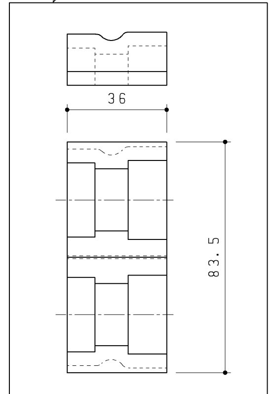
防露カバー（分岐金具部）
