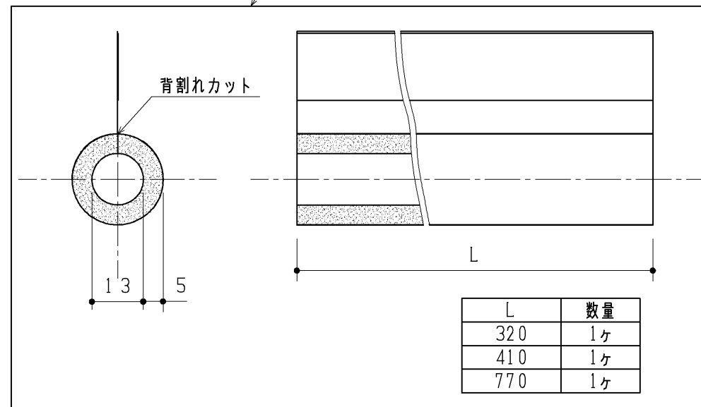
防露材 3ヶ
