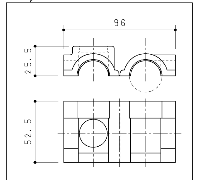
防露カバー（分岐金具部）
