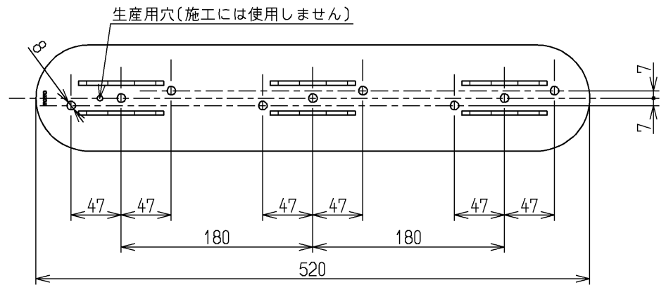
取付座詳細(1:5)
