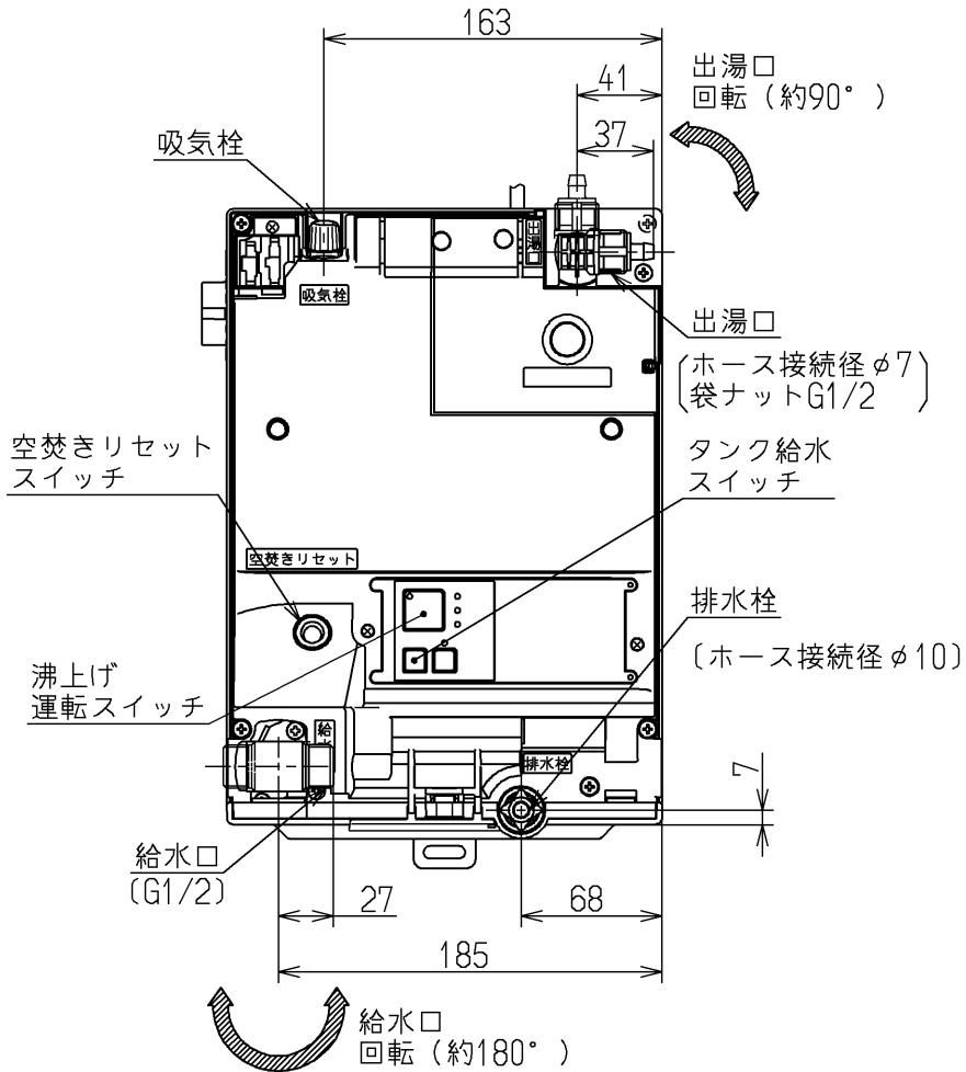
■化粧カバー取外図
