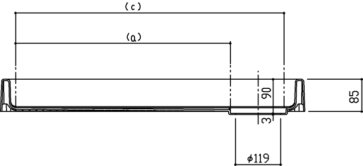
断面A-A
