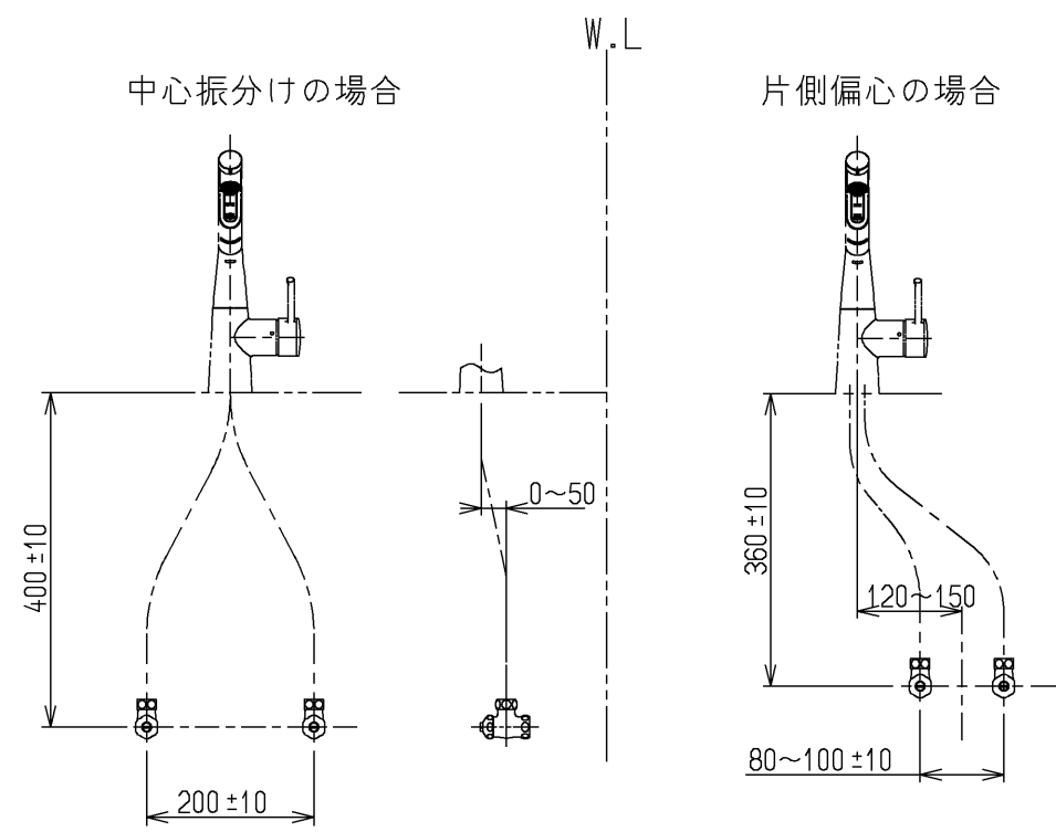
止水栓推奨取付位置
