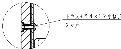
A部詳細 (S=1:2)
