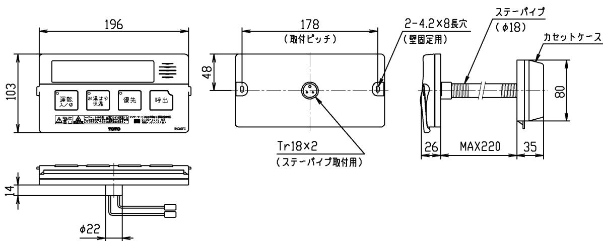
■浴室リモコン（別売品：RAC112FS）（1：5）
