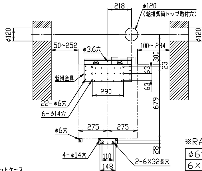
■壁取付位置（1：20）
