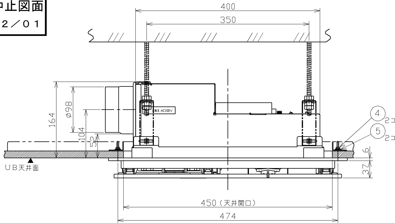
天井取付図
