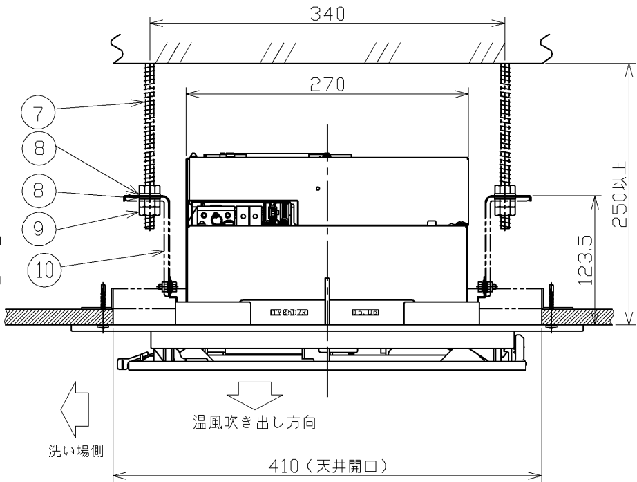
天井取付図
