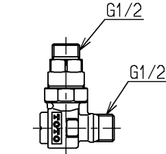
止水栓部 (2ヶ)
