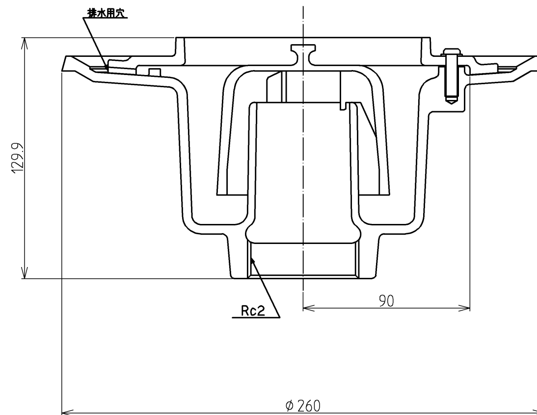
A-A'断面
