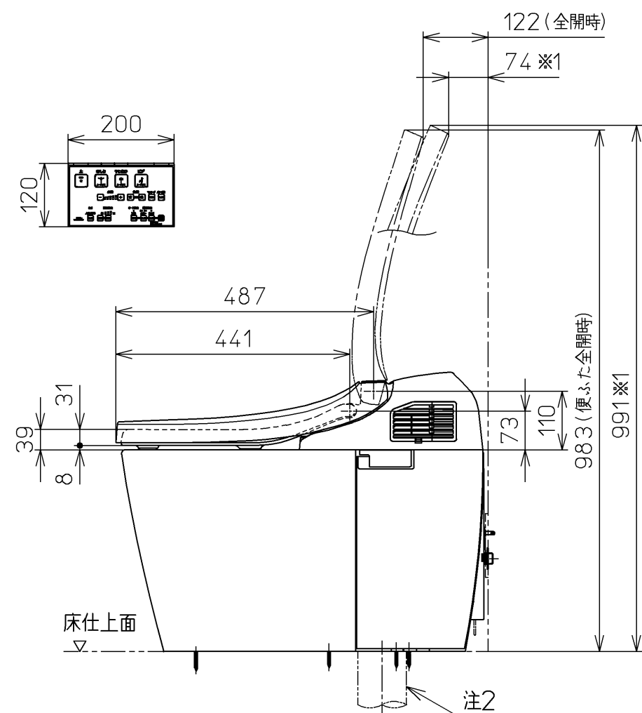
床給水仕様の場合
