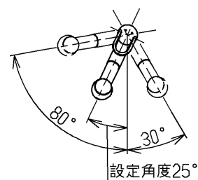
右配置図
