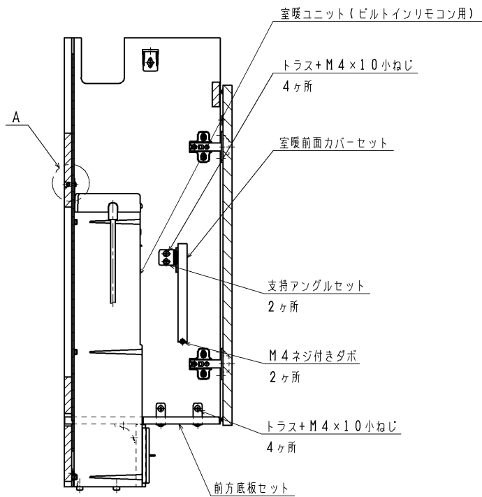
室暖ユニット固定詳細
