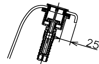
断面B-B(1:5)
