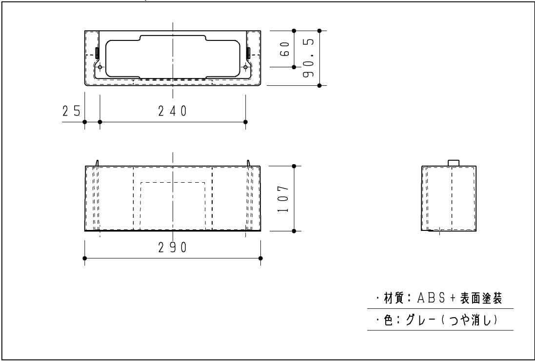
配管カバー(蹴込み) 1ヶ
